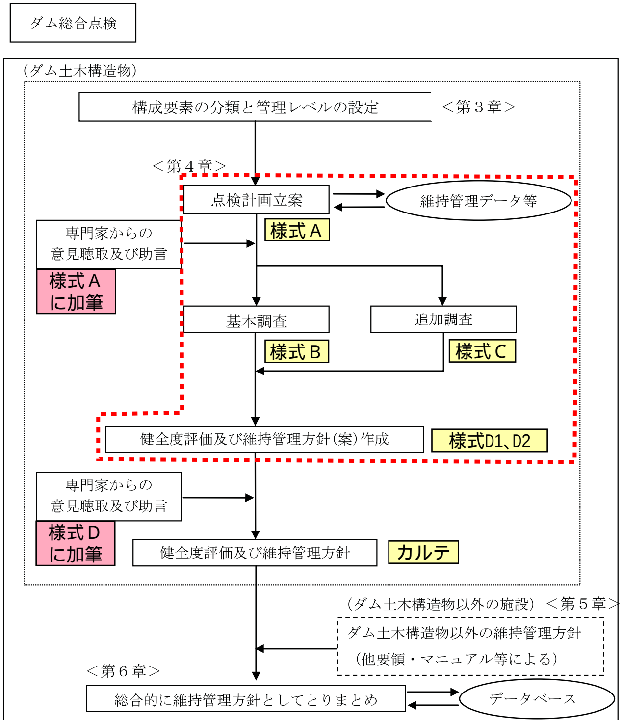
図 1.2-3 ダム総合点検の基本フロー
